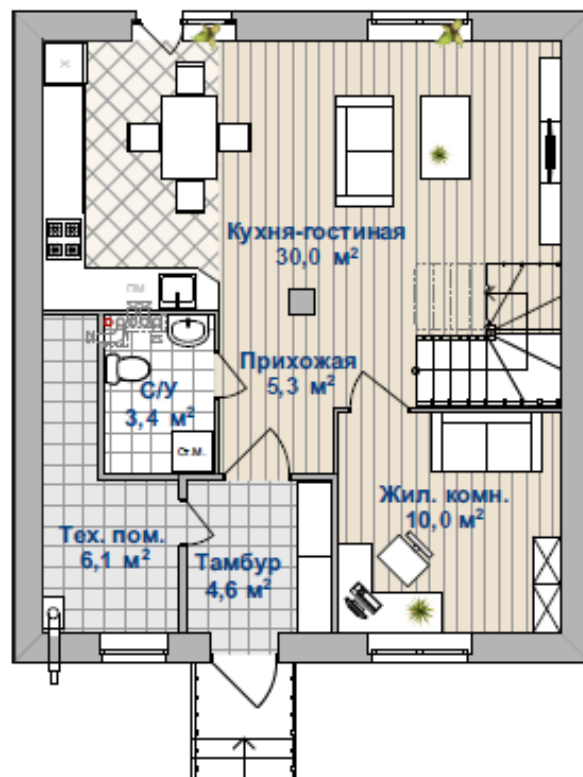
ПЛАН 1 ЭТАЖА
